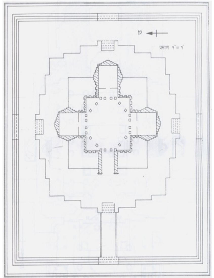
२४. अन्वा, शिवमंदिरों तलविन्यास, जि. जालना
