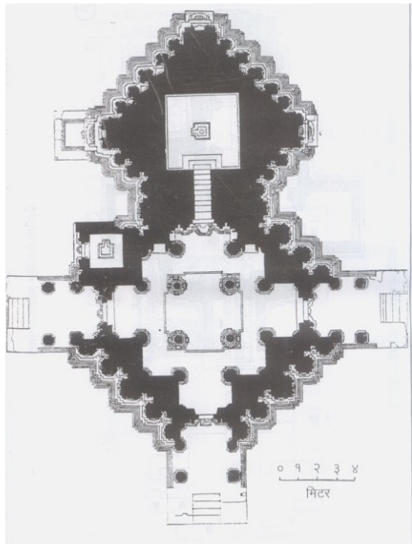
१८. अंबरनाथ शिवमंदिरांतलविन्यास, जि. ठाणे
