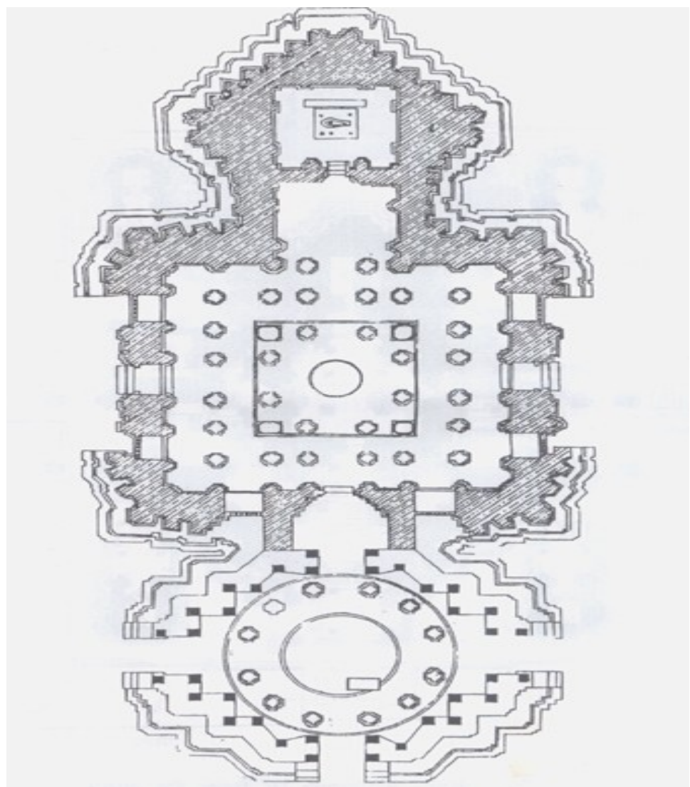
२०. कोप्पेश्वर मंदिरांतलविन्यास, ता. शिरोळ, जि. कोल्हापूर
