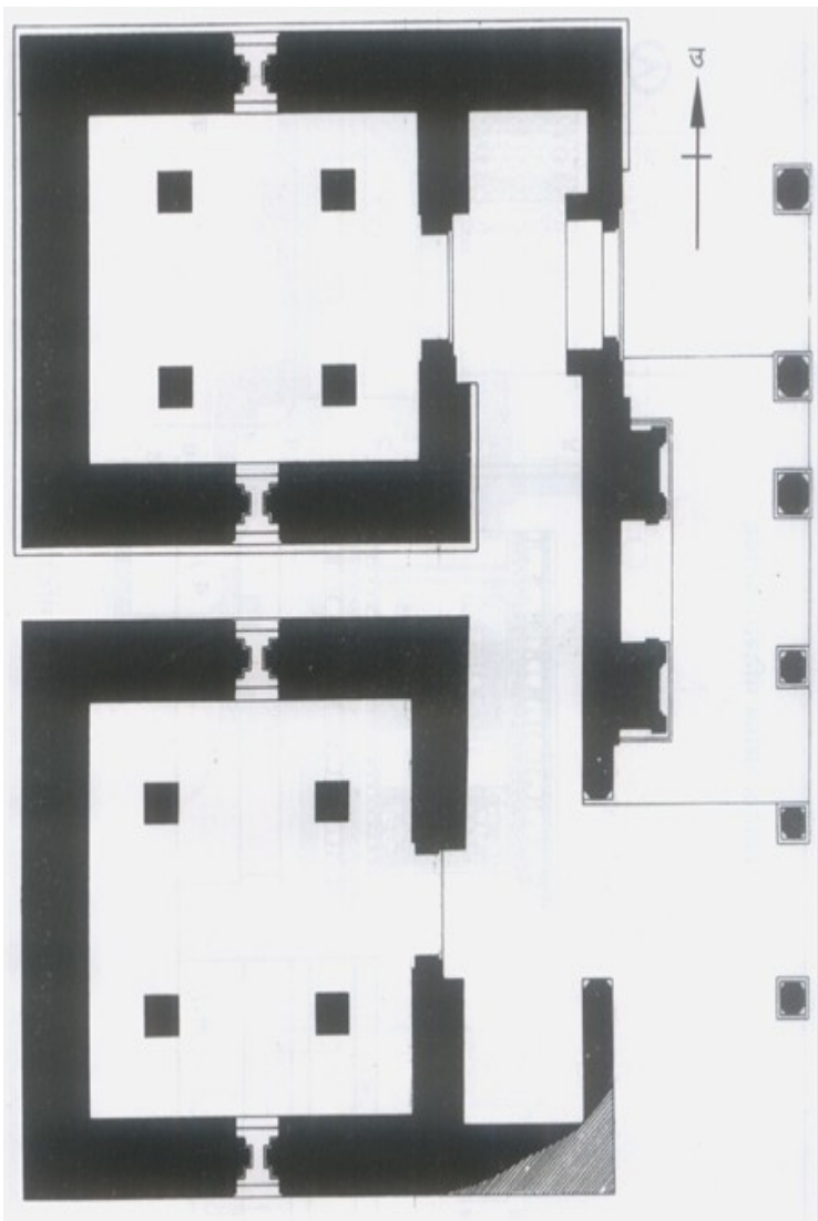
१५. भोगराम मंदिरोंतलविन्यास, रामटेक, जि. नागपूर
