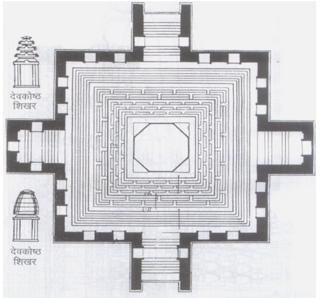
३२. जागजी येथील बारवोतलविन्यास, जि. उस्मानाबाद
