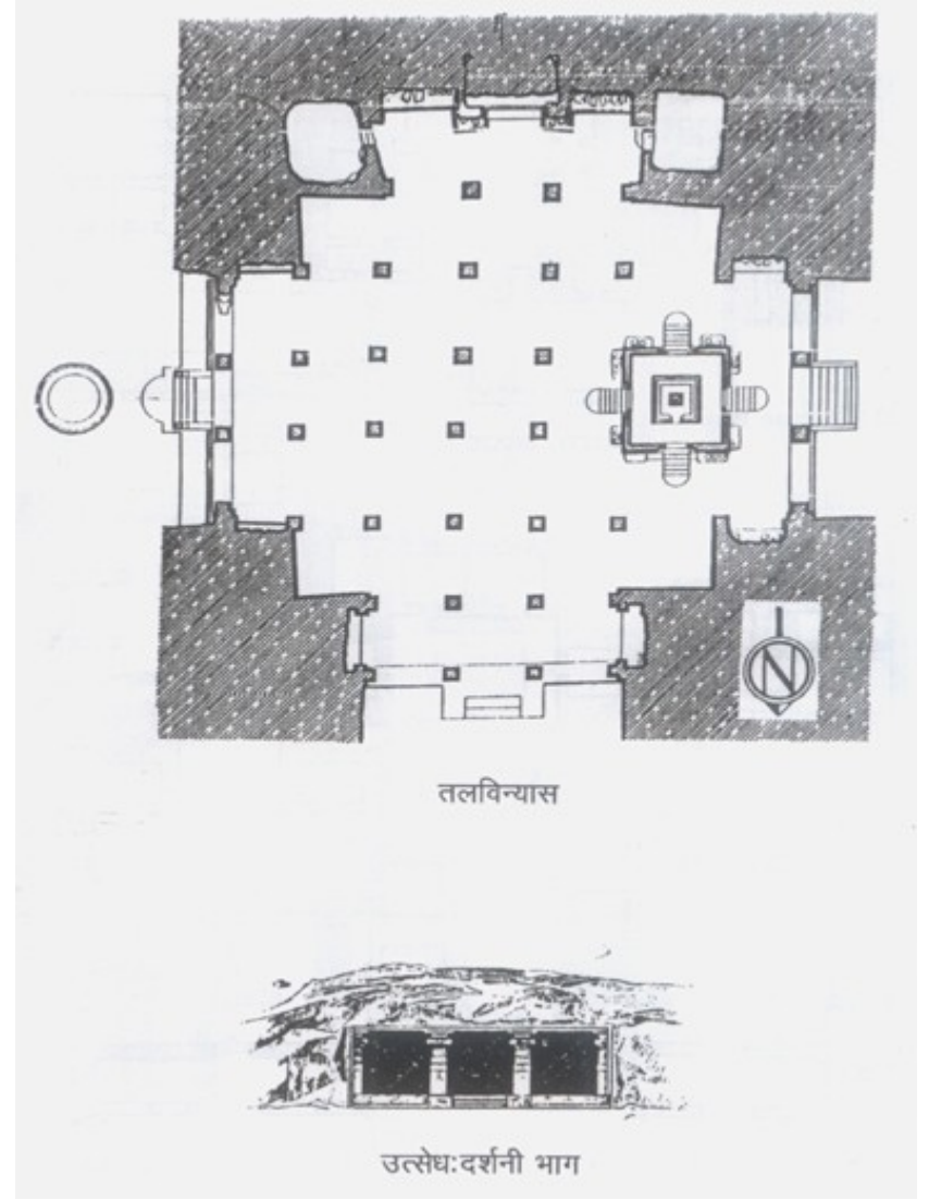
१०. घारापुरी लेणी क्र. १० तलविन्यास, ता. उरण, जि. रायगड
