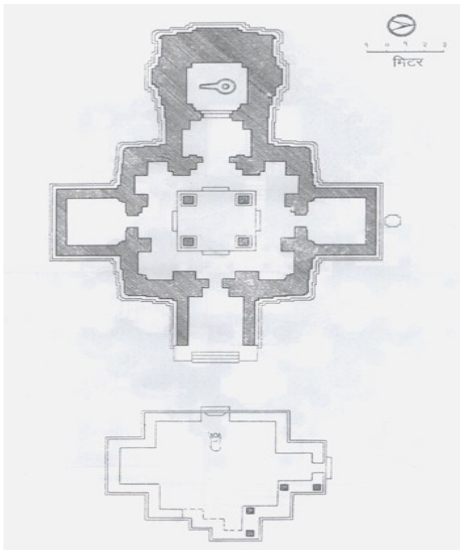
१७. मार्कंड ऋषी मंदिर व नंदिमंडप, मार्कंडीतलविन्यास, ता.चामोर्शी, जि. गडचिरोली
