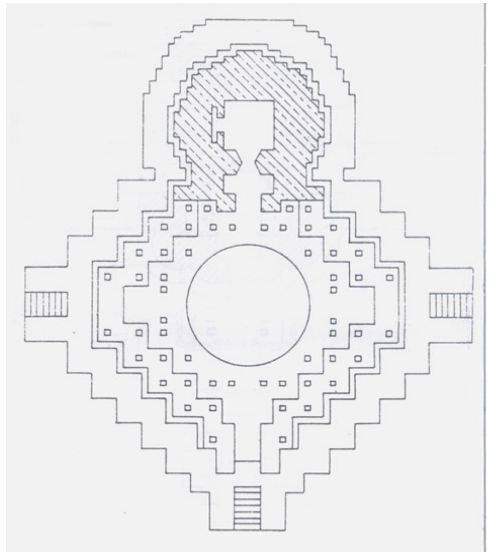
२४. अन्वा, शिवमंदिरों तलविन्यास, जि. जालना
