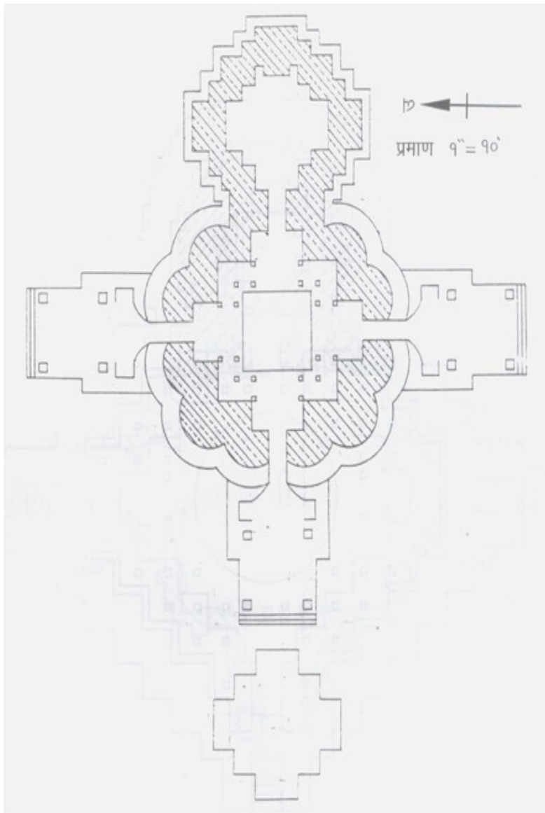
२३. औंढा, नागनाथ मंदिरों तलविन्यास, ता. औंढा नागनाथ, जि.परभणी
