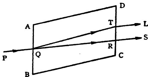
চিত্র ৩৬ দ্বৈত প্রতিসরণ।
