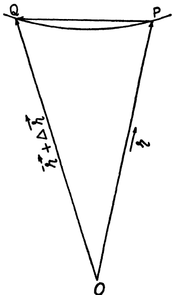
চিত্র 1'5—সরণ ভেক্টর
