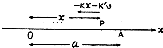
চিত্র 2.10—অবমানিত সমজস্য দোলন।
