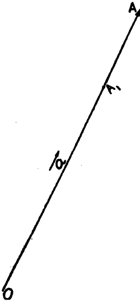
চিত্র 1.1 ভেক্টর \vec{a} পরিমাণ
