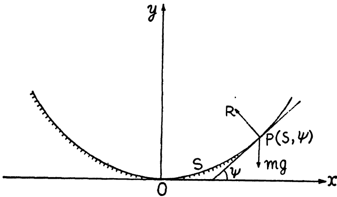
চিত্র 3.13—মসৃণ চক্রজের উপর মাধ্যাকর্ষণ-জনিত কণার গতি
