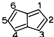
Pentalene
