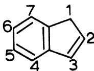
Indene
