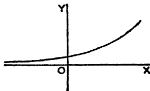
(ii) y = e^x .
